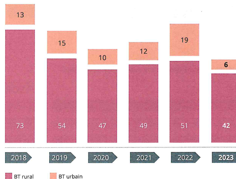
Évolution du nombre de départs BT mal alimentés par zone
